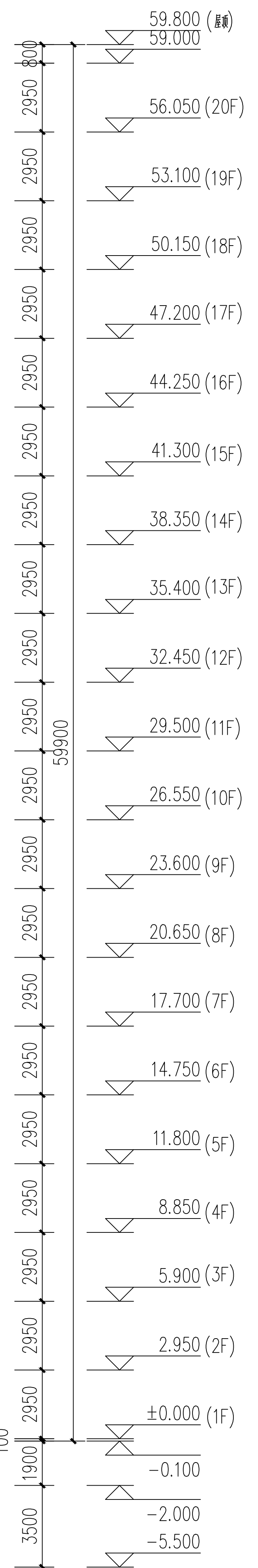
20层剖面图 (变更剖面)
